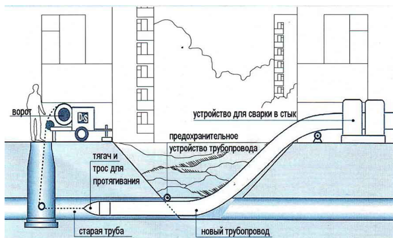
Рис. 1. Схема релайнинга трубопроводов.
