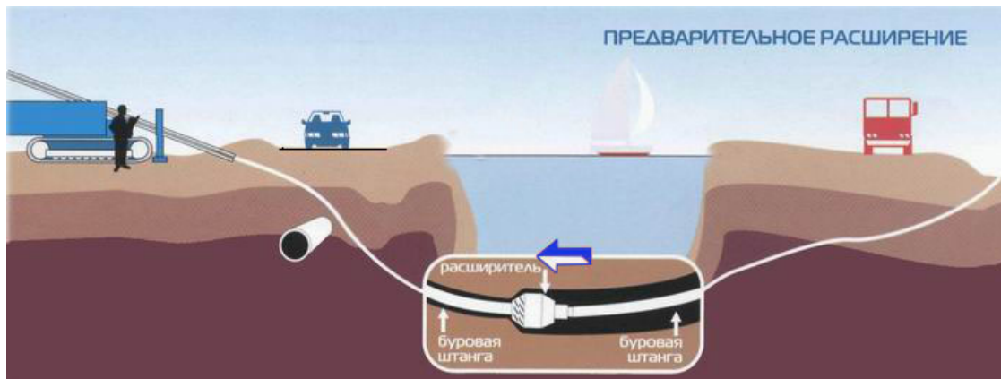
Рис. 6. Схема расширения скважины
