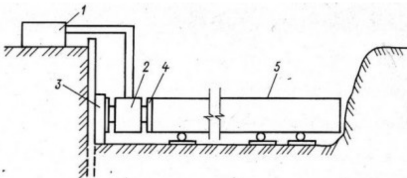
Рис. 3.24. Схема выполнения продавливания 1 — масляный насос; 2 — гидравлический домкрат; 3 — опорная конструкция; 4 — опорная плита; 5 — продавливаемая труба
