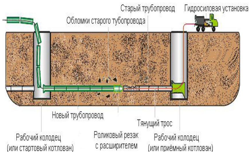
Рис. 2. Схема реновации трубопровода.
