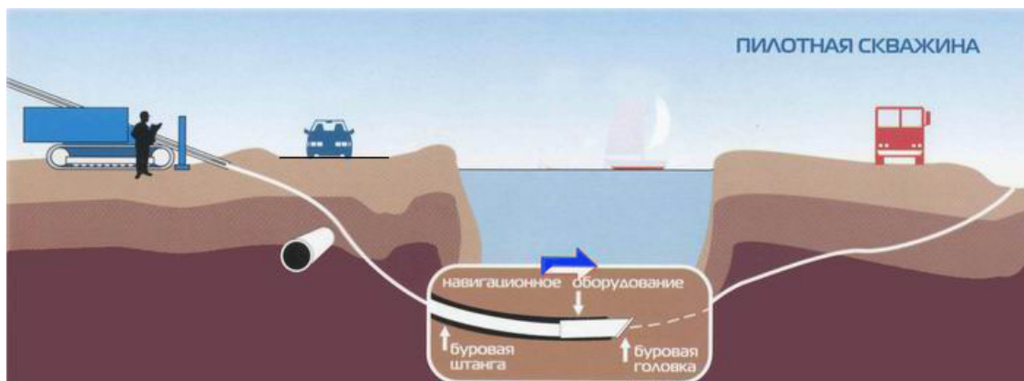
Рис. 5. Схема прокладки пилотной скважины
