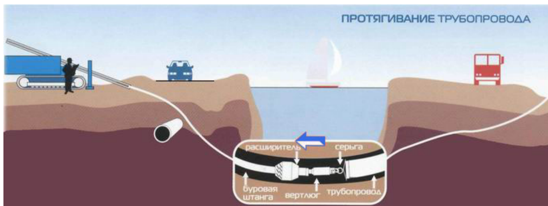
Рис. 7. Схема протягивания трубопровода
