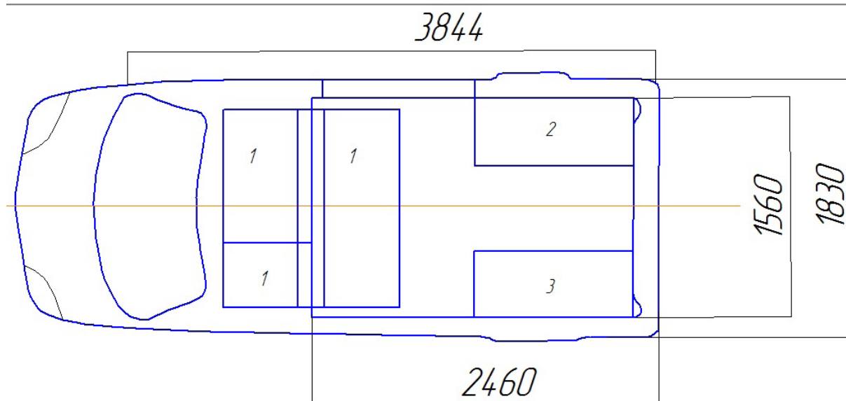
Рис. 2. Примерная компоновка специализированного автомобиля: 1 – раздвижные сиденья, 2 – места под оборудование (холодильник, генератор, сейф), 3 – места под ящики и клетку для собаки)
