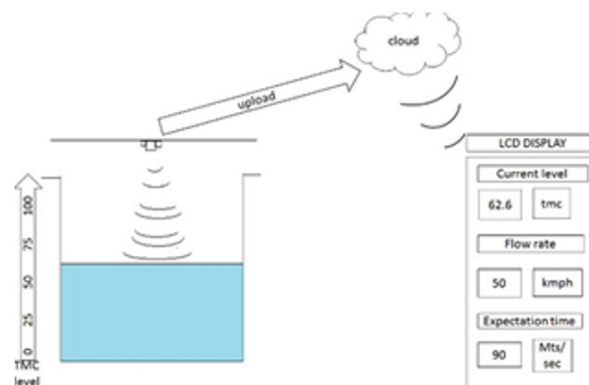
Рисунок 8 – Схема построения дистанционного мониторинга
