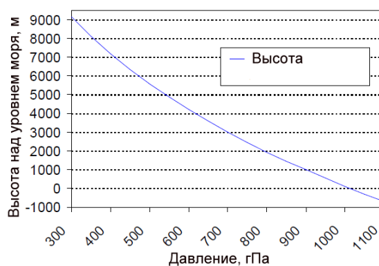
Рисунок 1. Зависимость высоты от атмосферного давления
