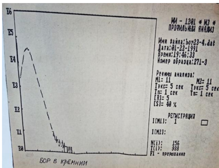
Рис. 1. Профиль распределения концентрации атомов бора по глубине образца монокристаллического кремния.
