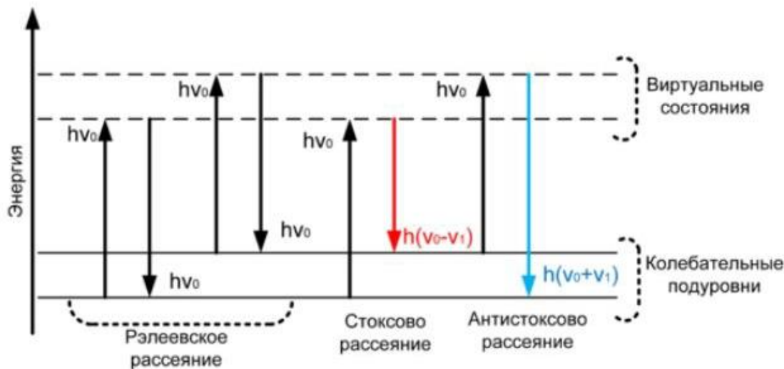
Рис.2. Иллюстрация квантового объяснения – эффекта Рамана.
